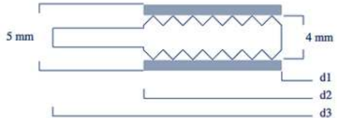
Kammprofildichtung nach EN 12560-6 für Flansche gemäß EN 1759-1
