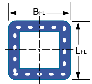
Flansch 2
